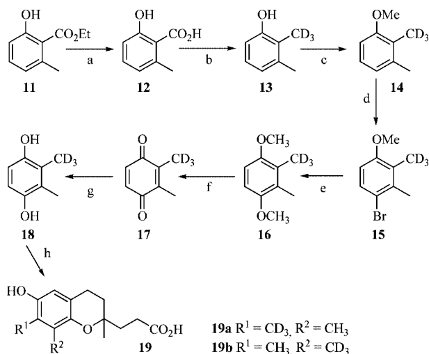
Scheme 2. a) \text{KOH} , \text{H}_2\text{O}/\text{MeOH} , 2:1, 50\text{ }^\circ\text{C} , 6 h, 94%; b) \text{ClCO}_2\text{Et} , \text{Et}_3\text{N} , 0\text{ }^\circ\text{C} , 2 h, then \text{NaBD}_4 , 8 equiv., \text{D}_2\text{O}/\text{THF} , 0\text{ }^\circ\text{C} , 3 h, 71%; c) \text{NaH} , \text{DMF} then \text{MeI} , 3 h, 89%; d) \text{BTMABr}_3 , \text{CH}_2\text{Cl}_2/\text{MeOH} , 1.5 h, 92%; e) \text{NaOCH}_3 , \text{CuI} , \text{MeOH}-\text{DMF} , reflux, 7 h, 88%; f) \text{CAN} , \text{CH}_3\text{CN}/\text{H}_2\text{O} , 20 min, 88%; g) \text{NaBH}_4 , \text{MeOH}/\text{H}_2\text{O} , 0\text{ }^\circ\text{C} , 20 min, 91%; h) 1 , \text{ZnCl}_2 , cat. \text{HCl}_{\text{conc}} , 1,4-dioxane, reflux 2 h, 43%.
